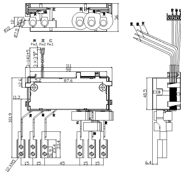
接线图 (wiring diagram)
