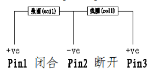
接线图 (wiring diagram)
